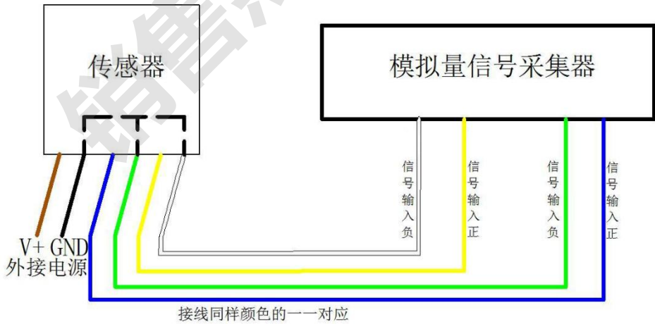
四线制接法示意图
