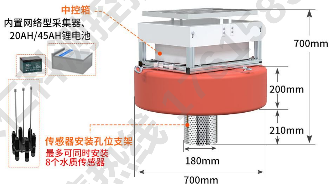
■ RS-SZJCZ-T3系列太阳能浮漂
